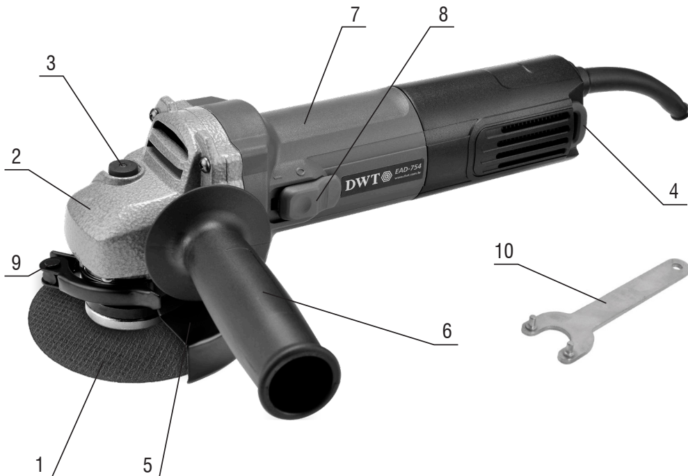
Figura 1 – Componentes da Esmerilhadeira
